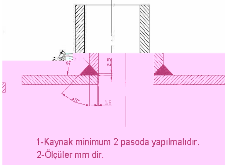
Şekil 8 Kurtağzı Kaynak Detay
